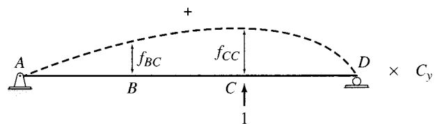
(d) Primary Beam Loaded with Redundant C_y
