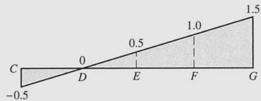
(d) Influence Line for B_y (kN/kN)
